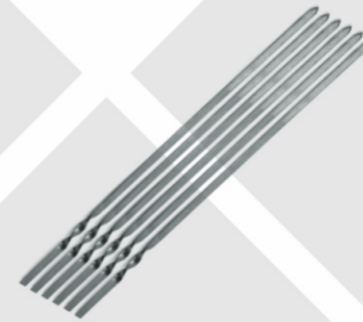
Шампуры Габаритные размеры Длина (мм): 500 Материал: нержавеющая сталь 2 мм.
