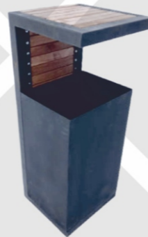
Урна уличная «Лофт» Габаритные размеры HxLxB (мм): 880x360x360 Емкость - 0,05 м3.
