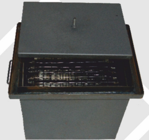
Устройство для копчения и сушки 170.000 Габаритные размеры НхLхВ (мм): 350x350x250 Масса: 11 кг. Материал корпуса: листовая сталь 1,5 мм. Материал решетки: нержавеющая сталь 2 мм. Двухъярусная с гидрозатвором
